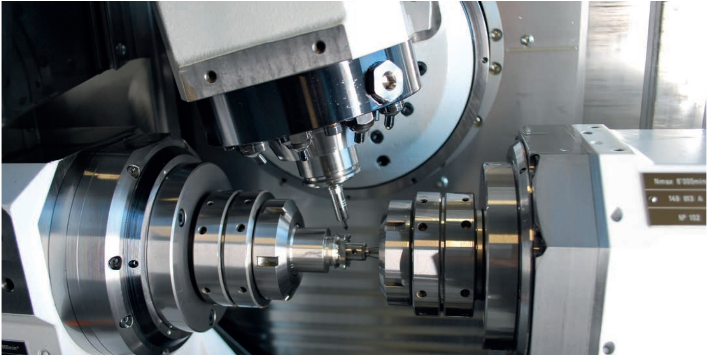
Usinage en simultané avec broche diviseur en axe A et contre-broche sur tourelle de reprise. Simultane Bearbeitung mit Teilspindel auf der A-Achse und Gegenspindel auf der Abgreifeinheit. Simultaneous machining with dividing spindle on the A-axis and counter-spindle on the backworking turret.
